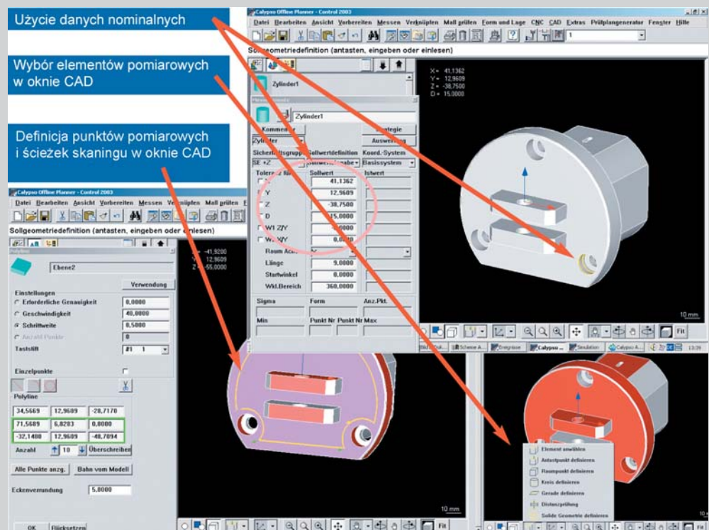
Rys. 1. Wykorzystanie danych CAD do definicji wymiaru nominalnego oraz generowania ścieżek skaningu
