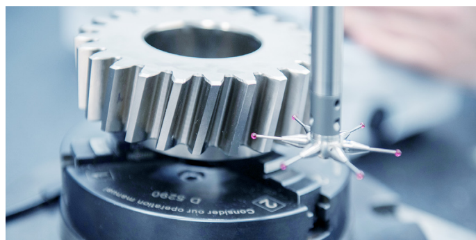
Pomiary kół zębanych
